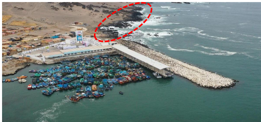
Figura N° 23: DPA Morro Sama, protegido mediante un rompeola (obra de abrigo artificial)
