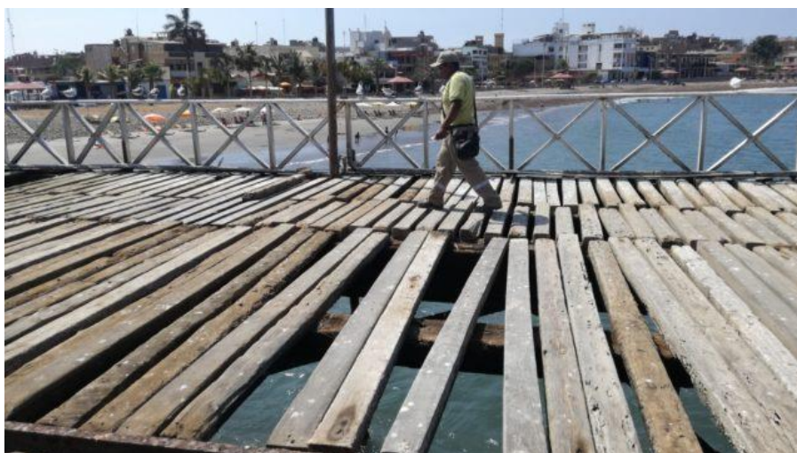
Figura N° 11: Sección de un muelle en situación de fragilidad
